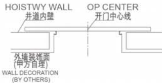
小门套示意图 SMALL JAMB SKETCH
