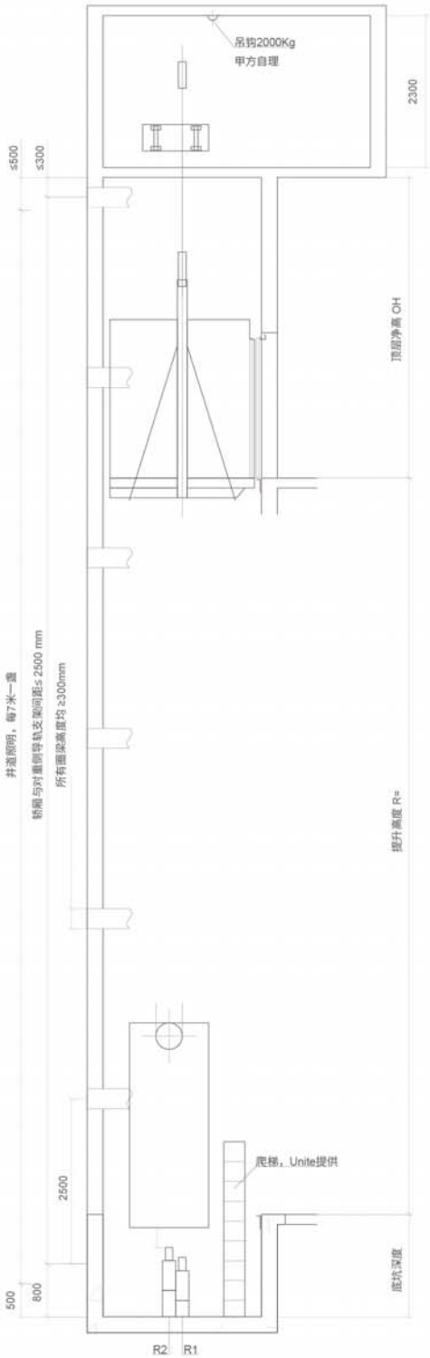
井道立剖面图 ELEVATION
