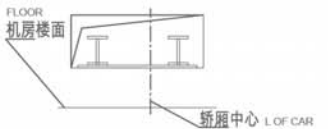
A-A承重孔 A-A BEARING HOLE
