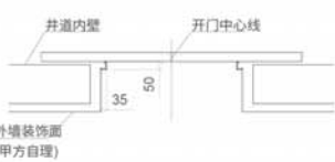
小门套示意图 SMALL JAMB SKETCH
