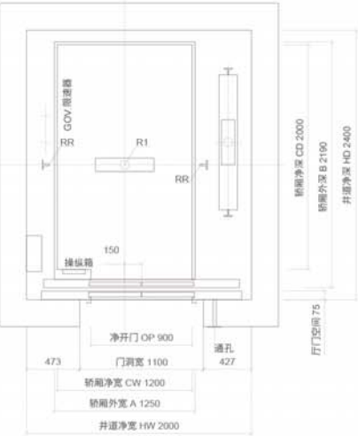
井道平面图 HOISTWAY PLAN
