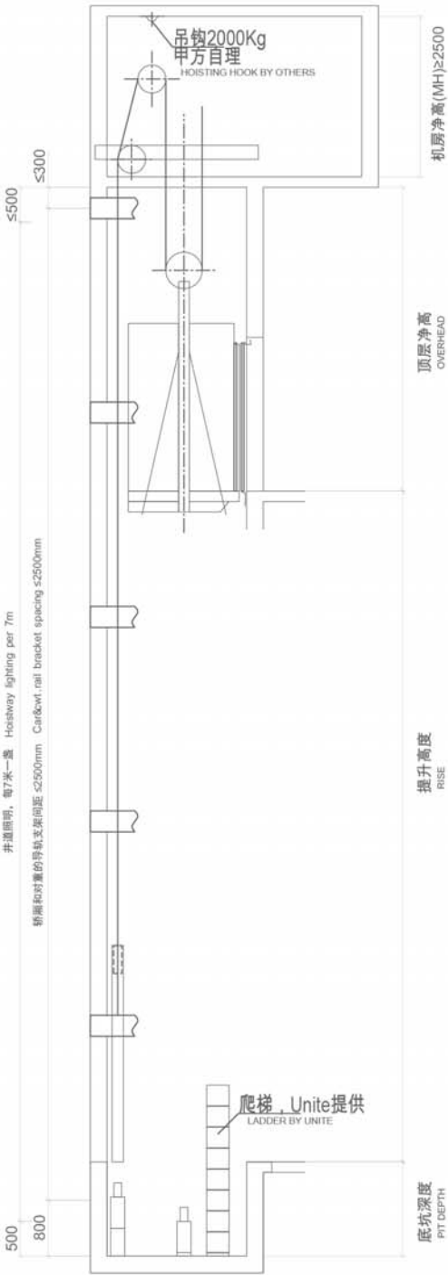
井道剖面图 ELEVATION
