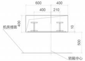
A-A承重孔 A-A BEARING HOLE
